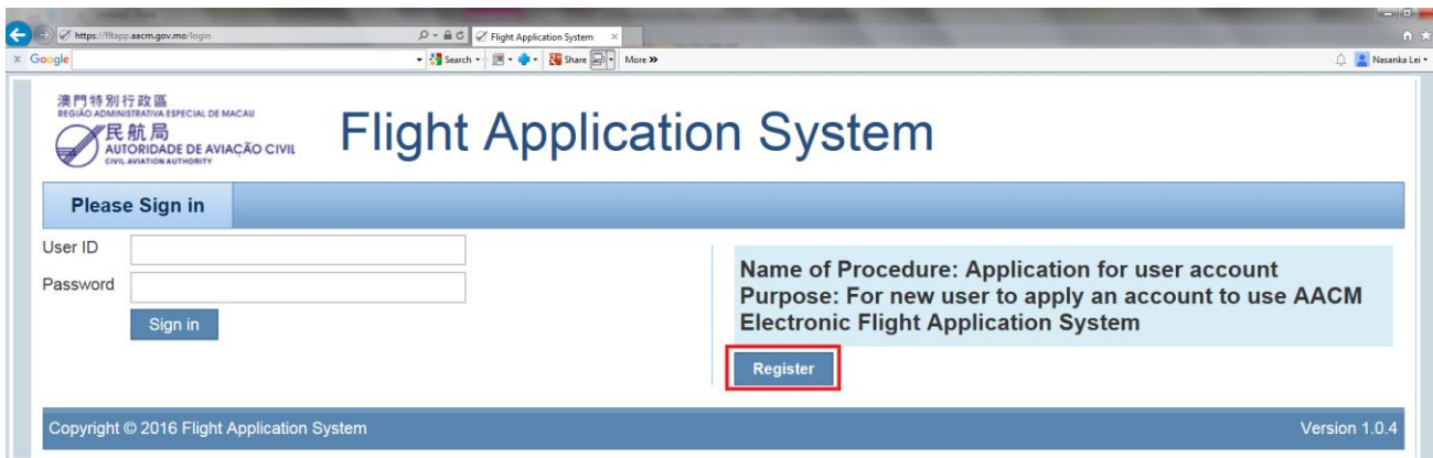
Login page
